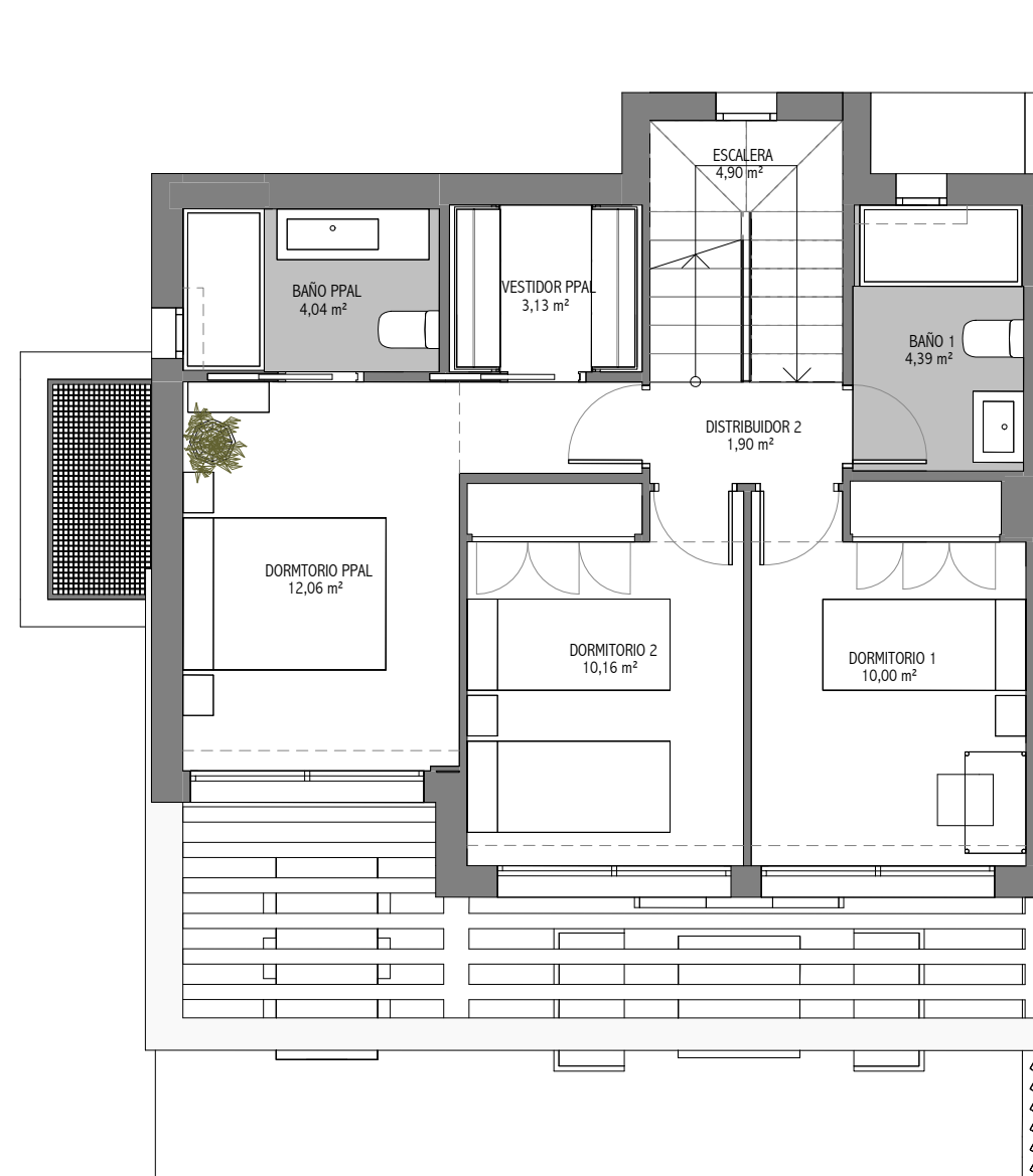
PLANTA ALTA 1:75
