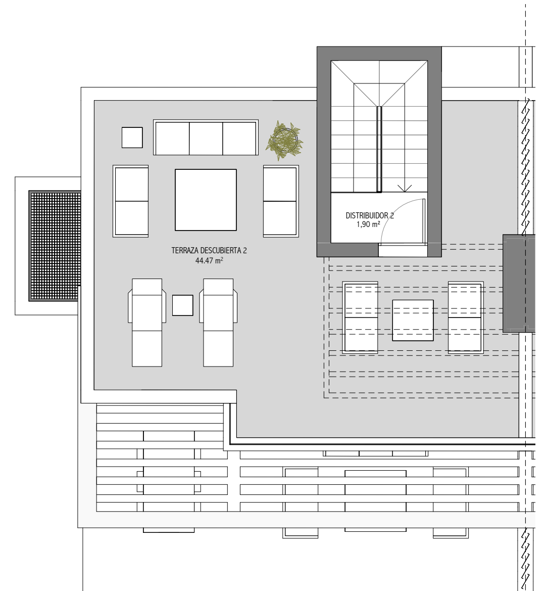
PLANTA SOLARIUM 1:75
