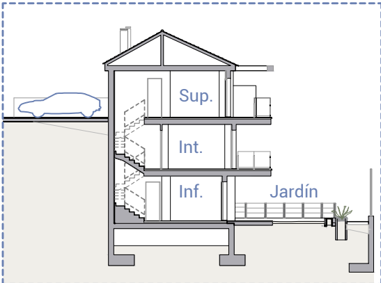
Sección / Section
