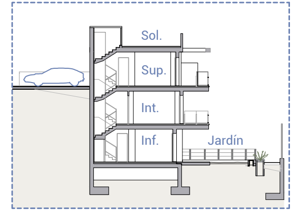
Sección / Section
