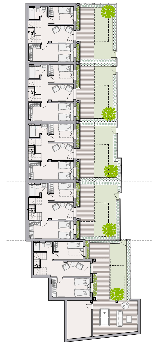
Planta / Floor Inferior
