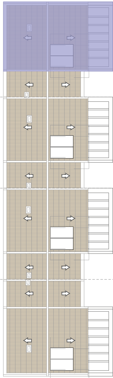
Cubierta / Roof
