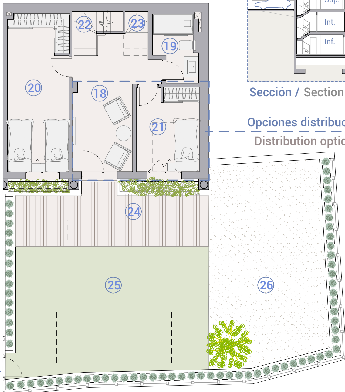
Opción 1: Bedroom + TV room Planta / Floor Inferior
