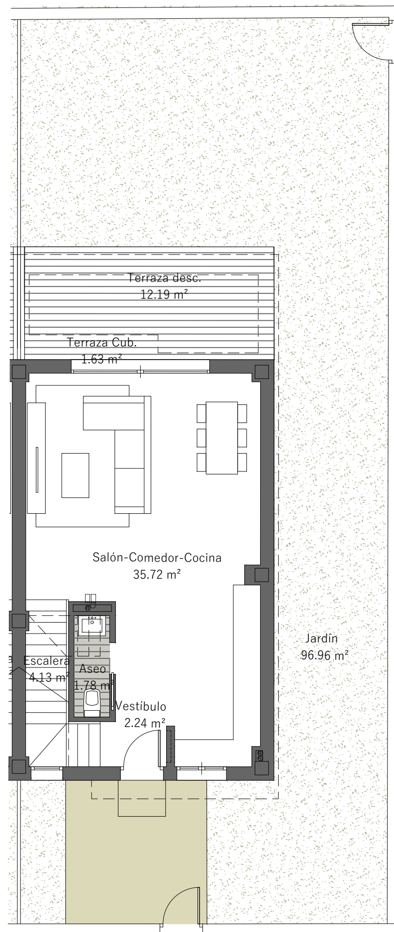
PLANTA BAJA
