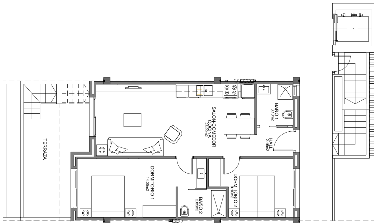
Planta Segunda
