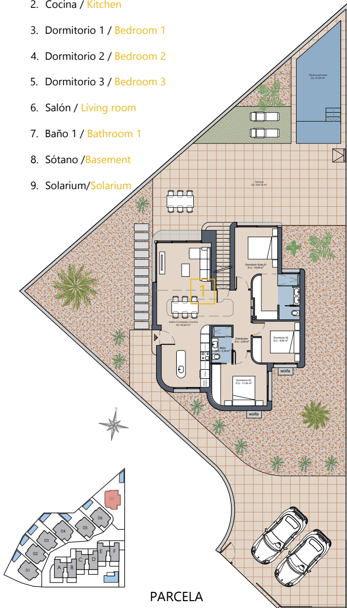
PLANTA BAJA
