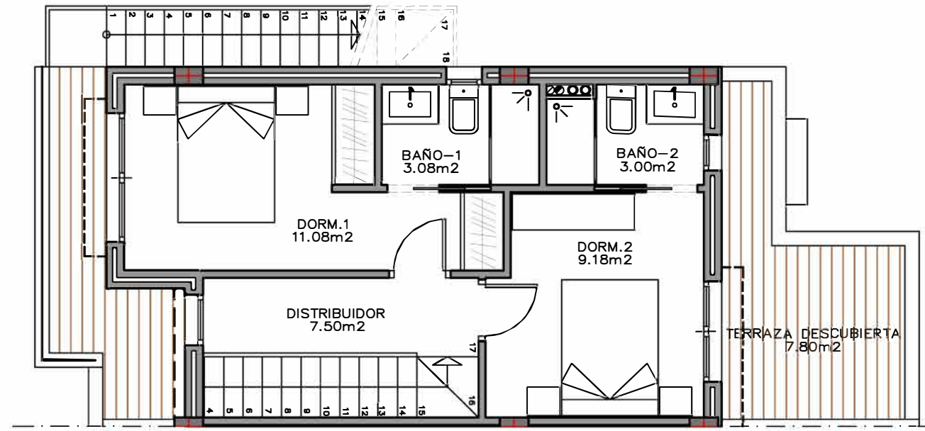
PLANTA PRIMERA
