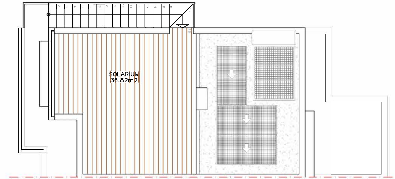
PLANTA CUBIERTAS
