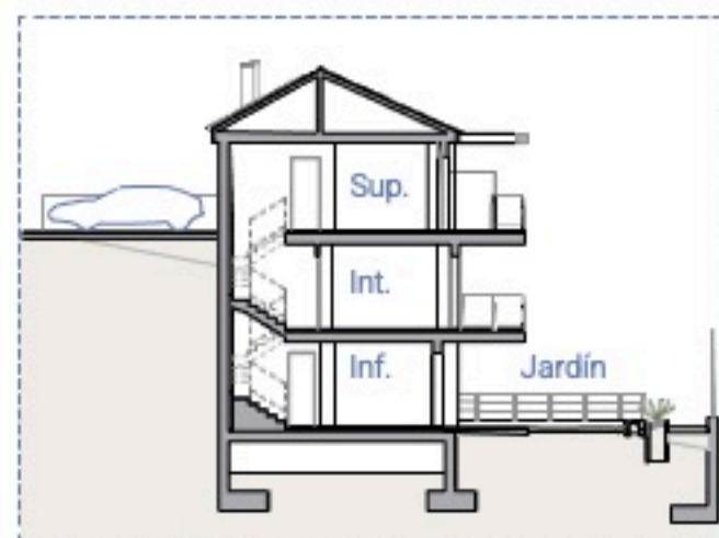
Sección / Section
