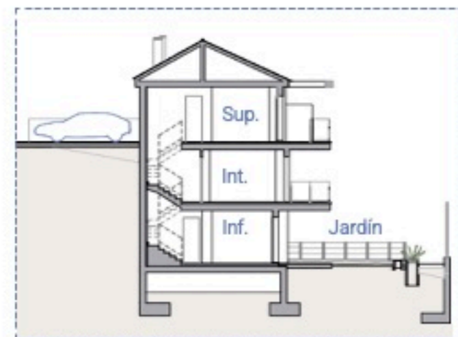
Sección / Section
