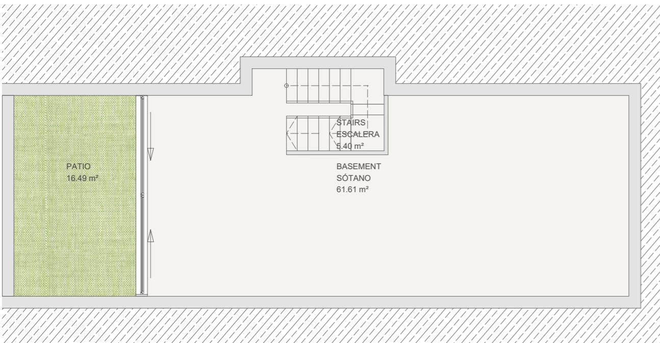
PLANTA SÓTANO
