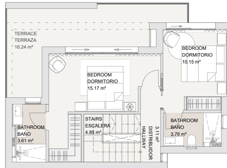
PLANTA SOLARIUM
