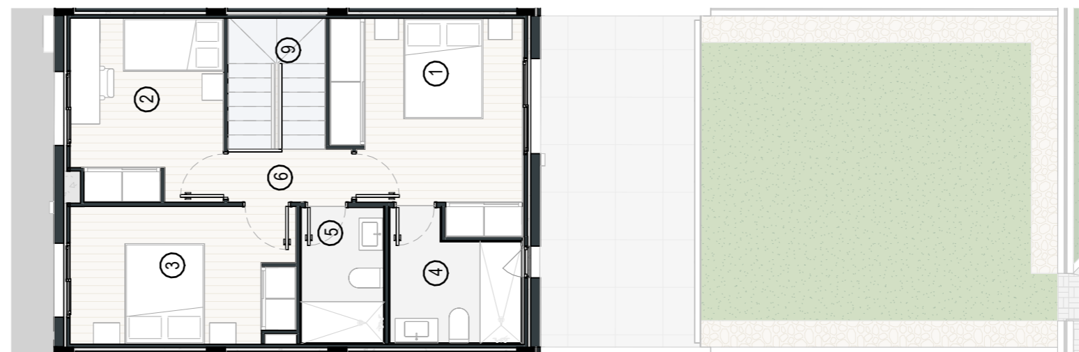
PLANTA PRIMERA
