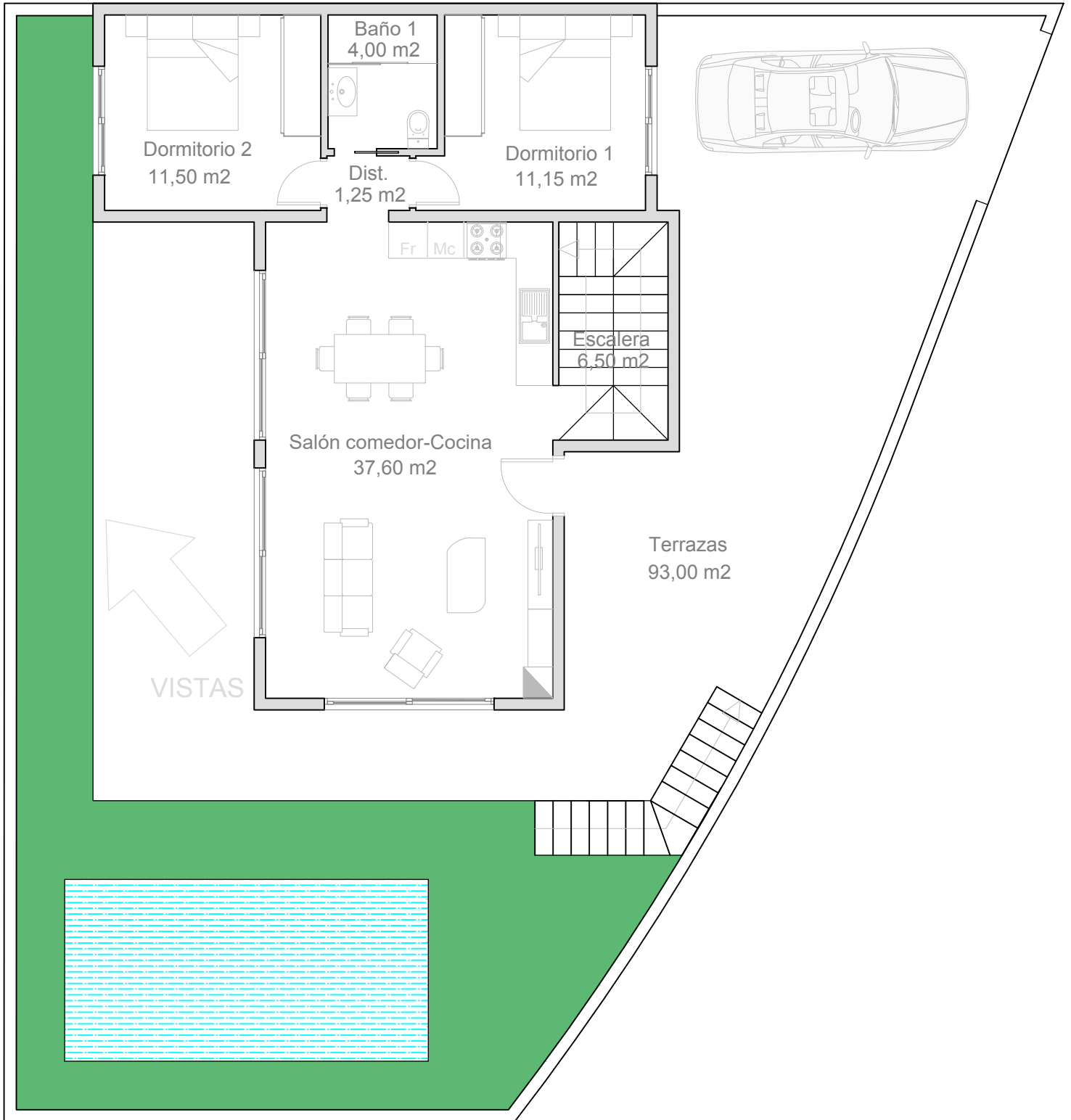
PLANTA INTERMEDIA
