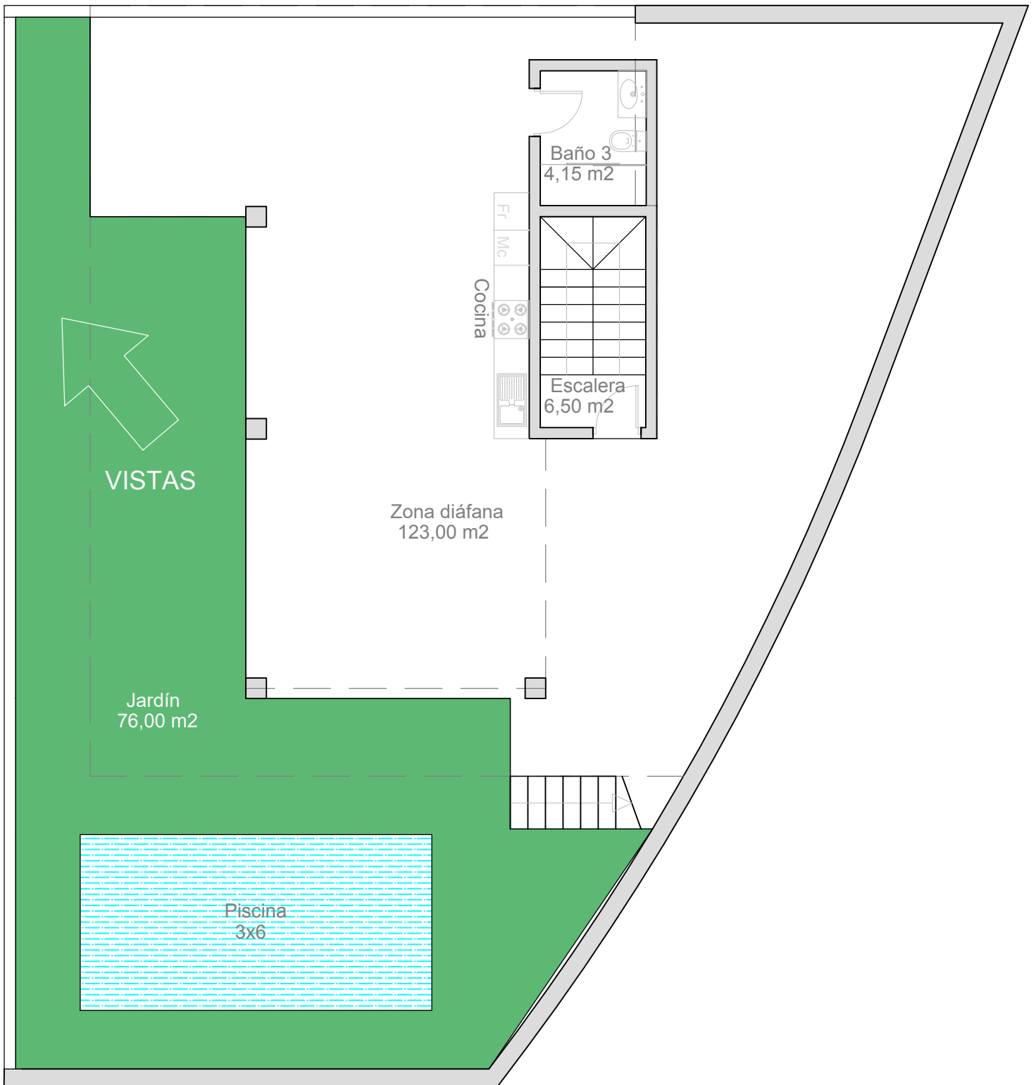
PLANTA BAJA
