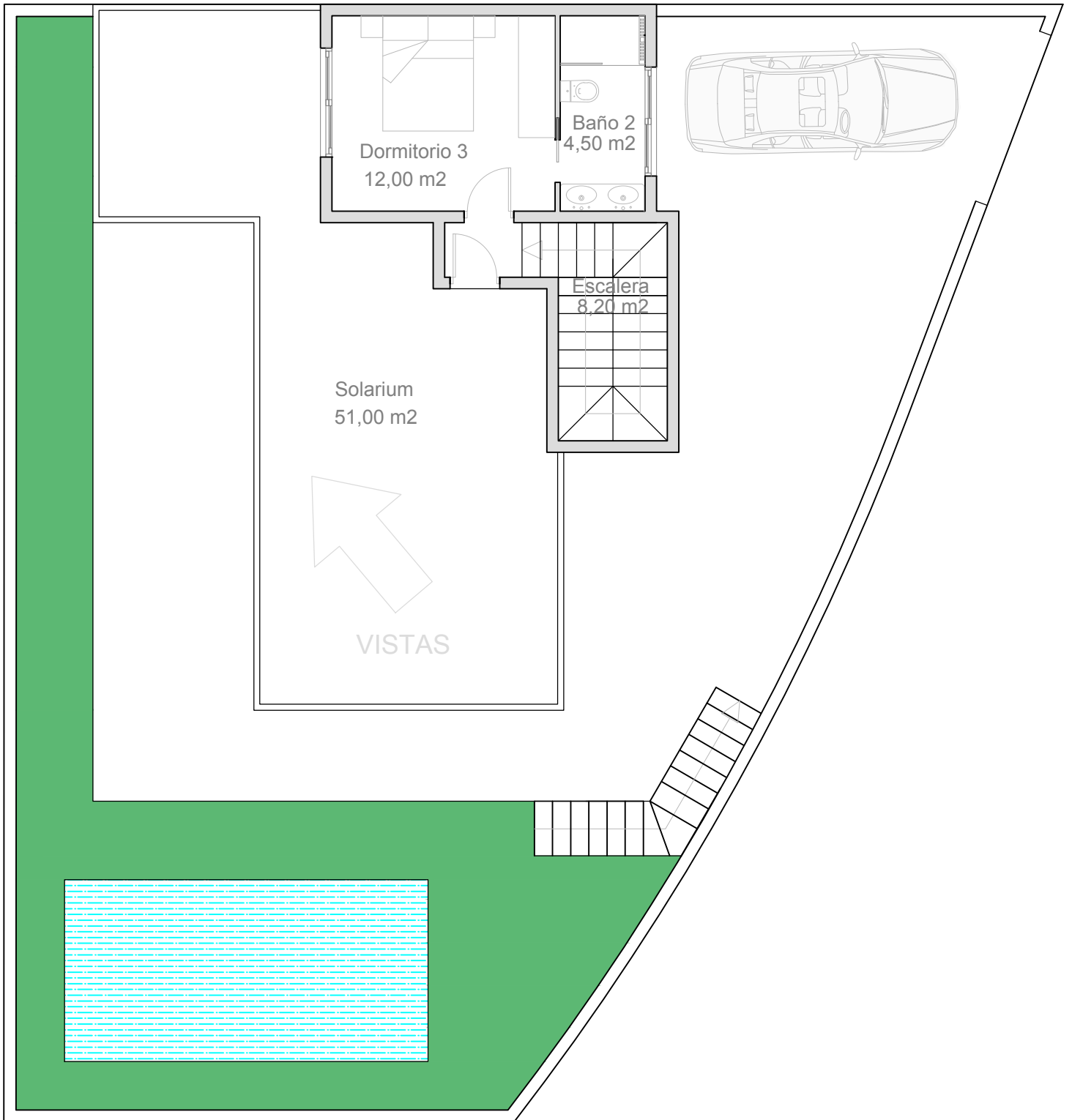
PLANTA ALTA
