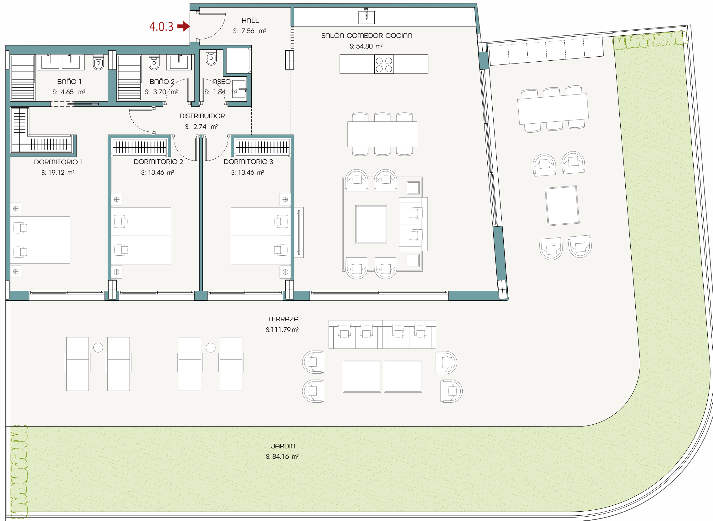
VIVIENDA 4.0.3 PORTAL 4 - PLANTA BAJA
