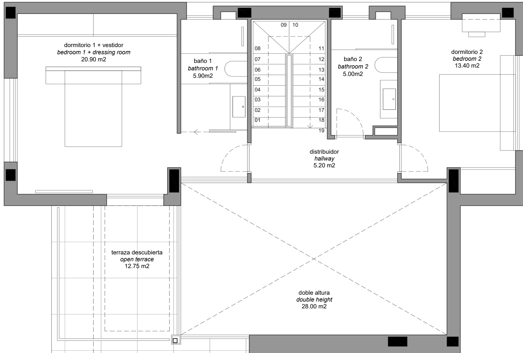
VIVIENDAS 3 Y 4 - PRIMERA PLANTA / HOUSE 3 & 4 FIRST FLOOR
