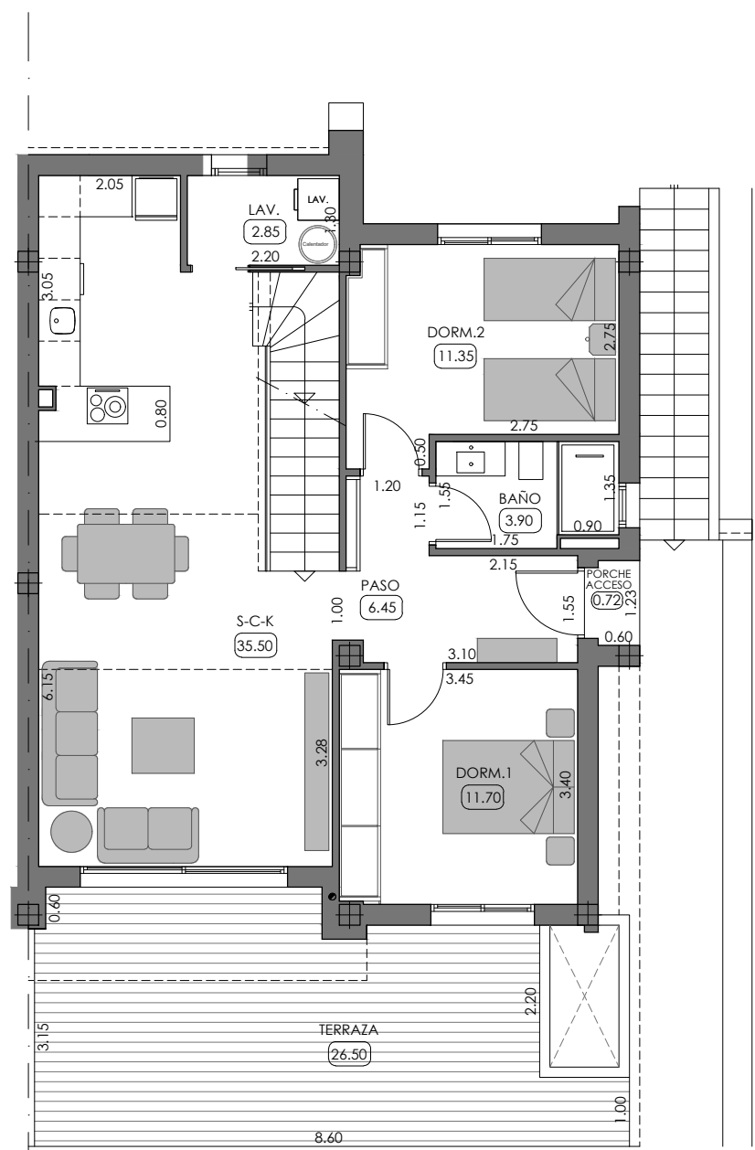
PLANTA BAJA
