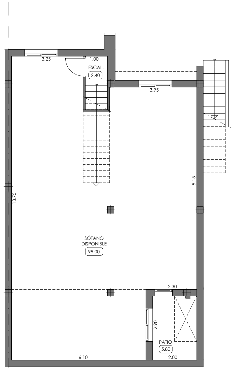
PLANTA SÓTANO
