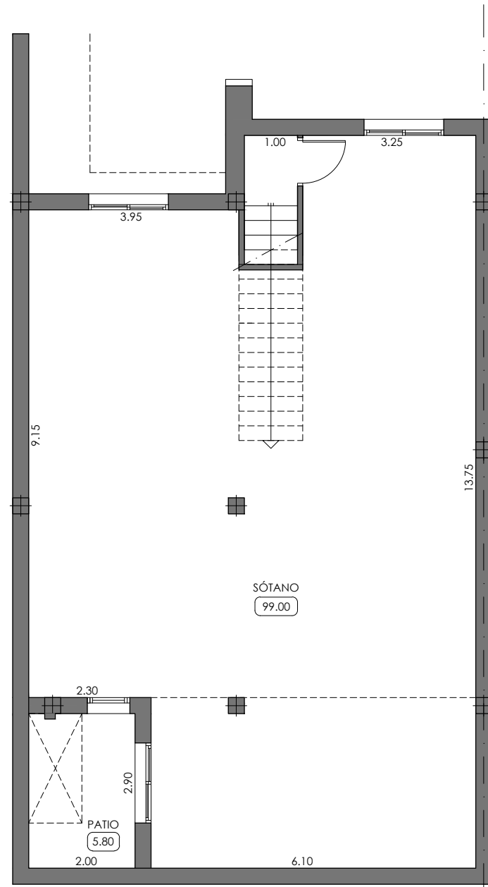
PLANTA SÓTANO
