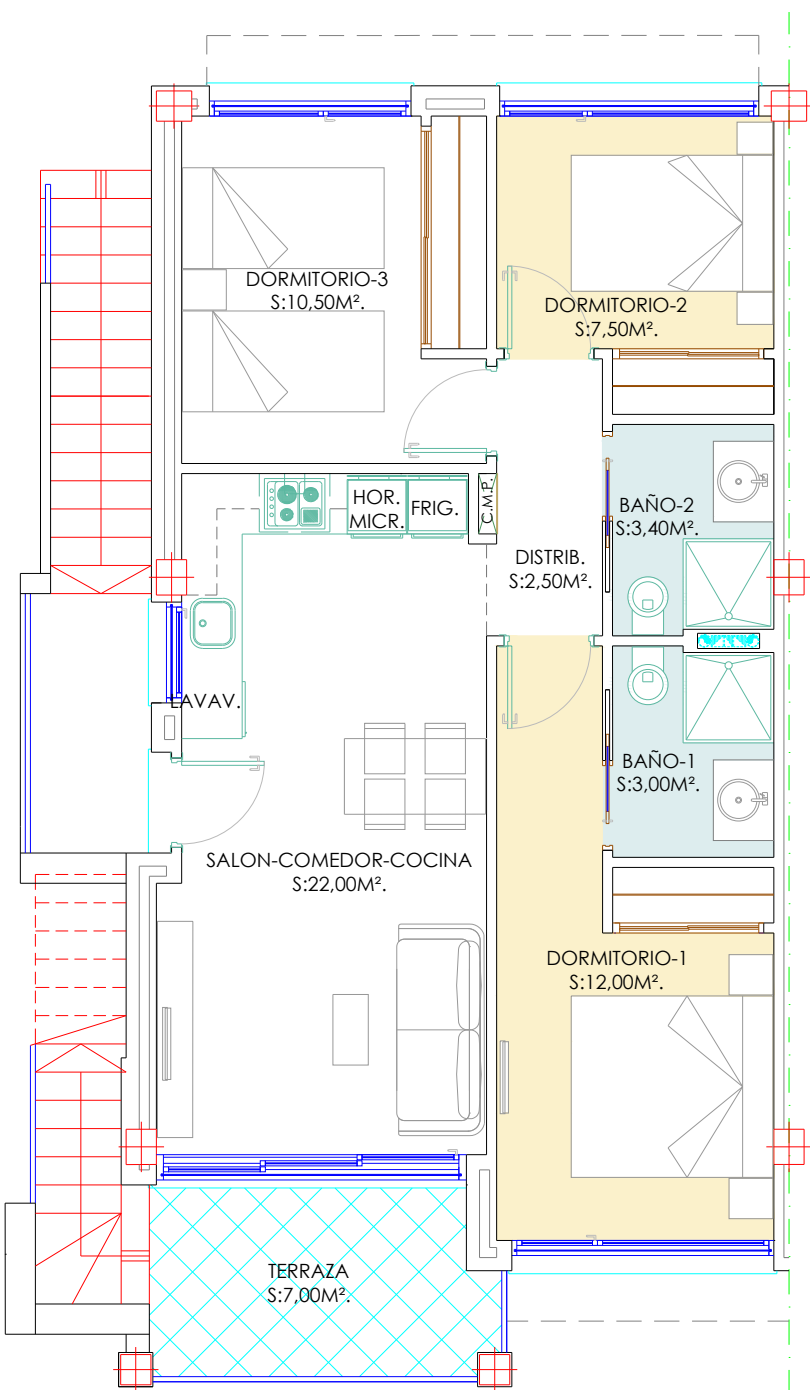
PLANTA PRIMERA
