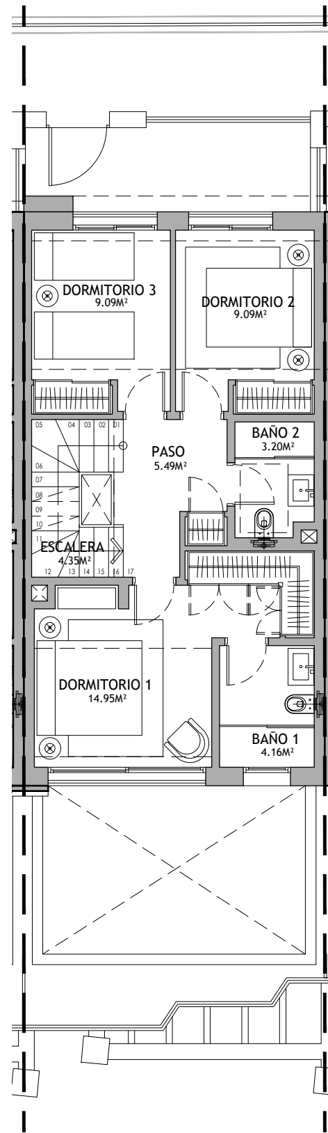
PLANTA ALTA
