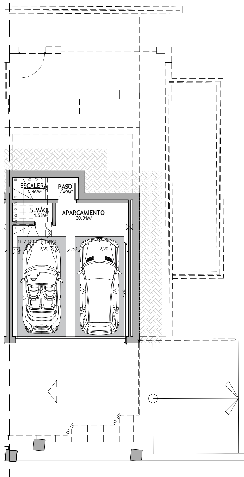
PLANTA SÓTANO T1.B V04
