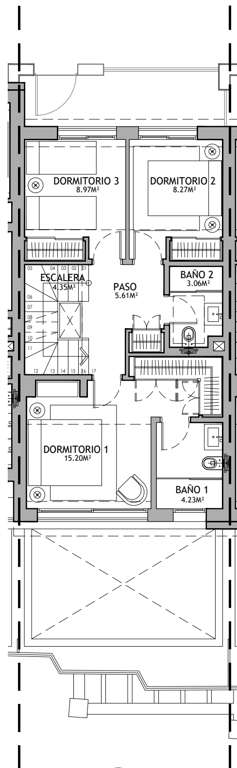
PLANTA ALTA
