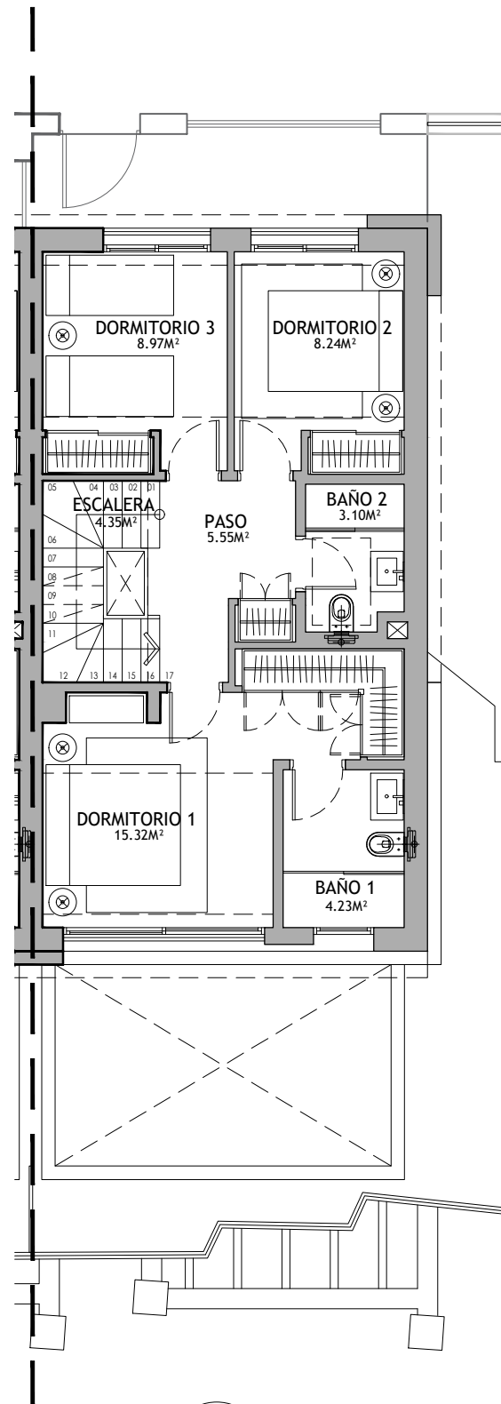
PLANTA ALTA T1-B V09
