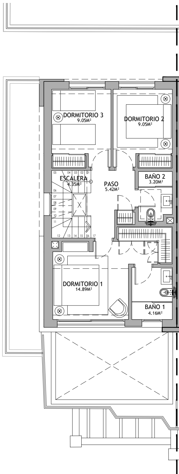
PLANTA ALTA
