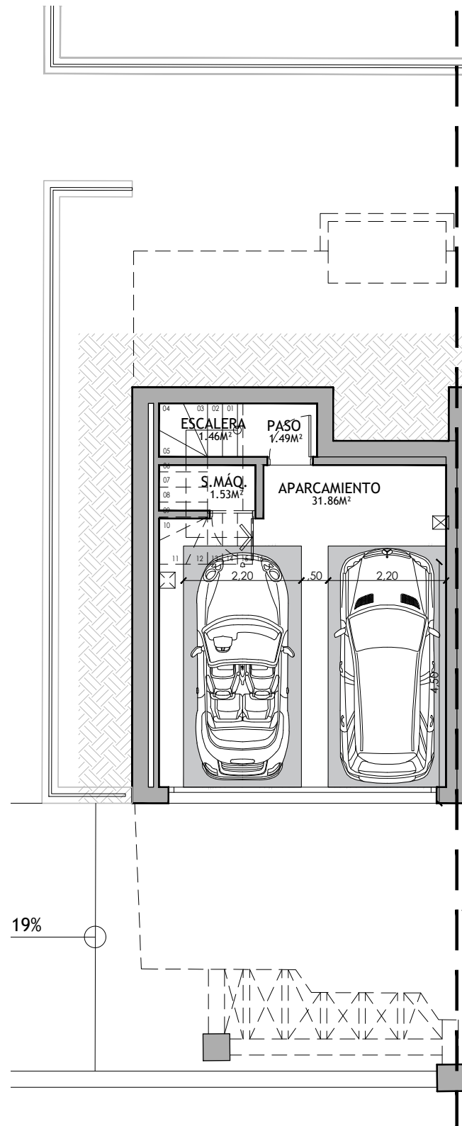
PLANTA SÓTANO T1-A V10
