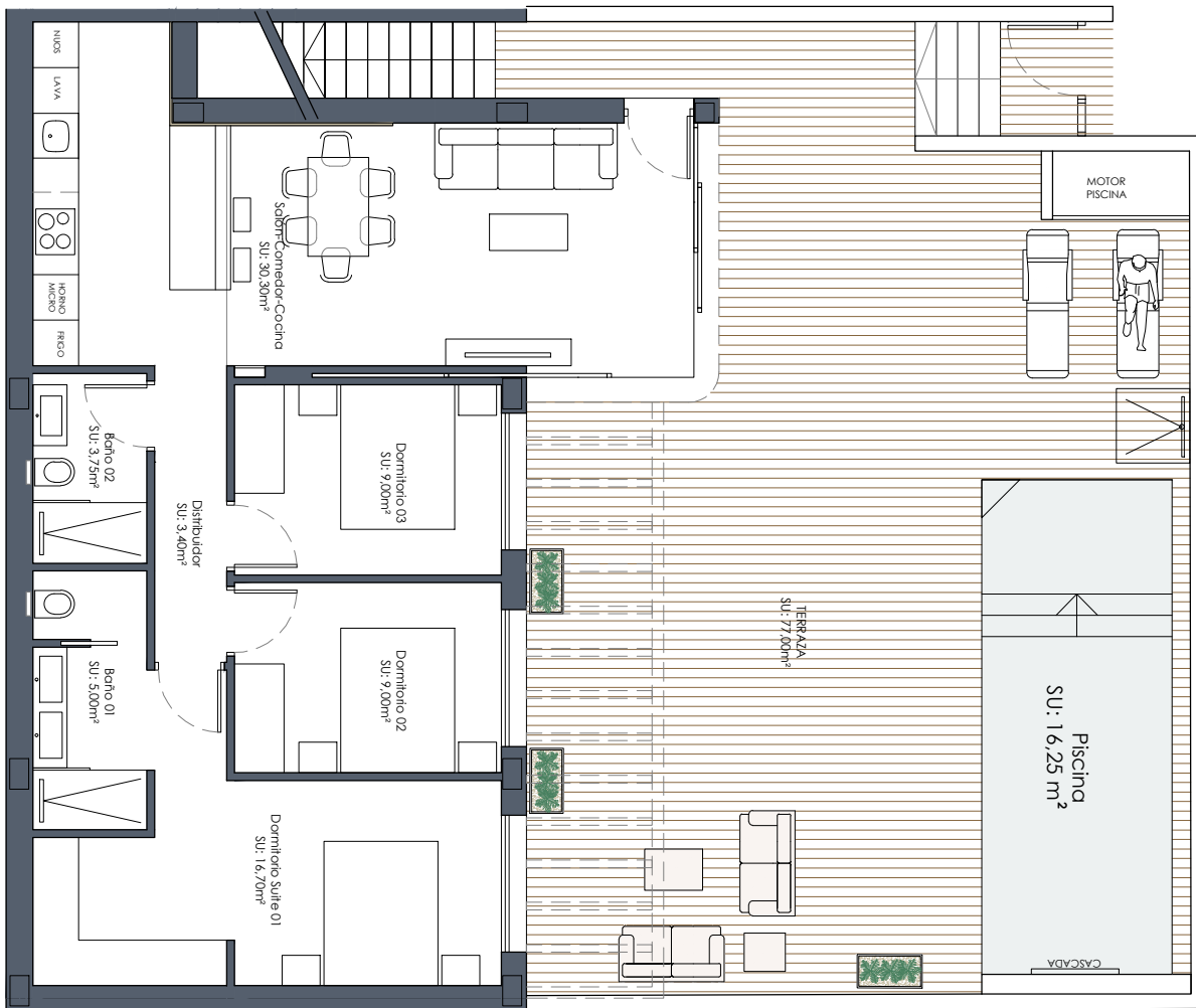
PLANTA BAJA
