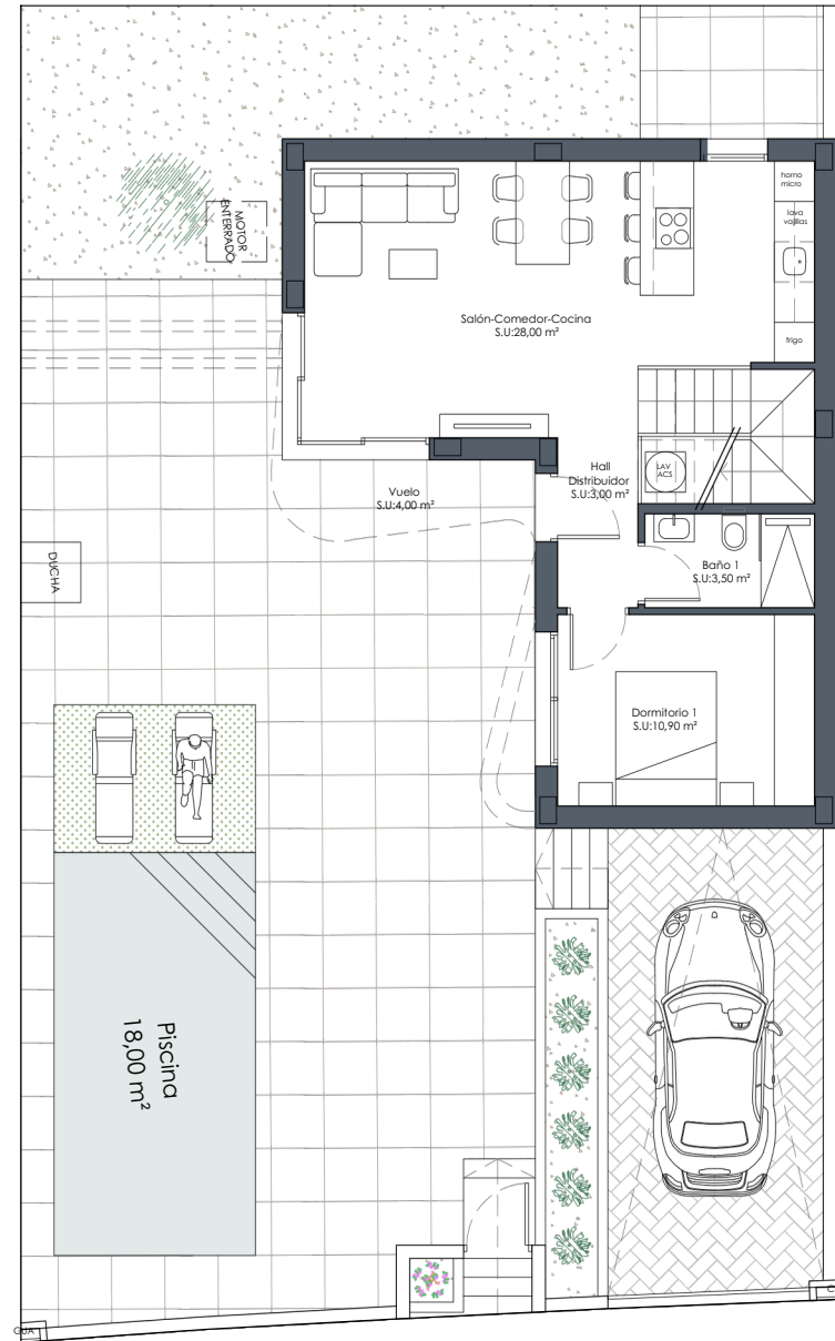
PLANTA BAJA
