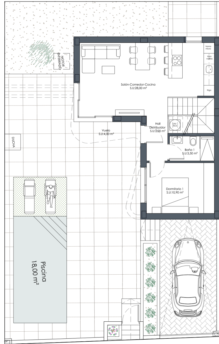
PLANTA BAJA
