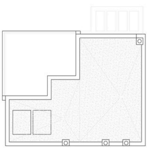
PLANTA CUBIERTA.
