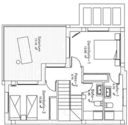
PLANTA PRIMERA.
