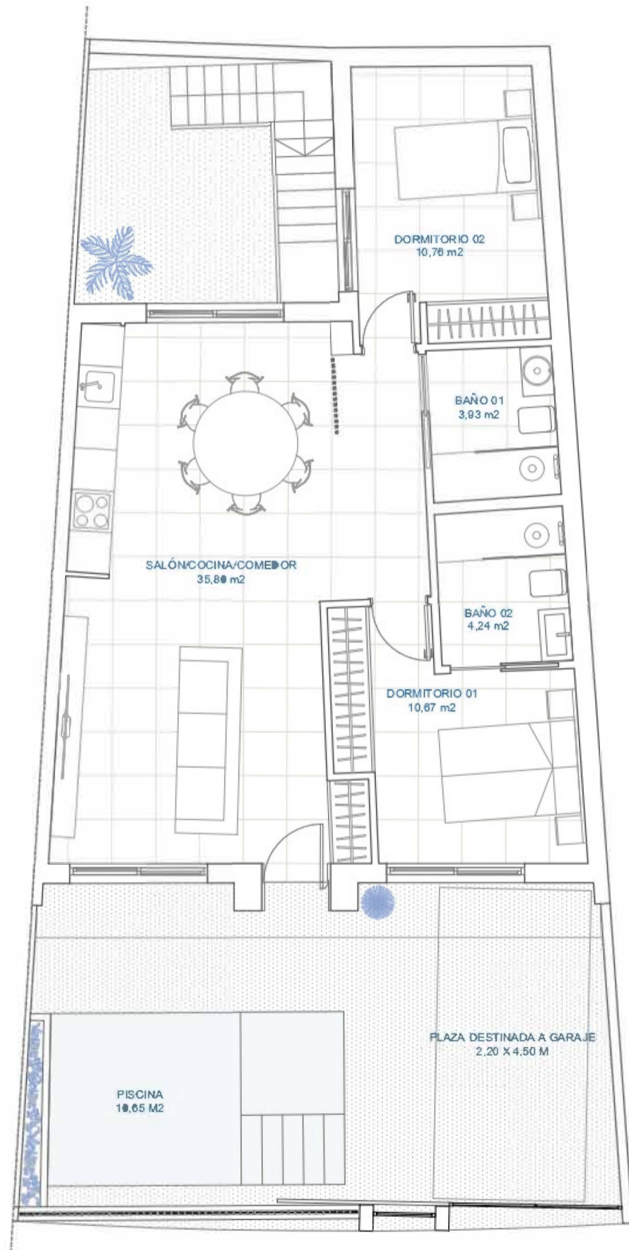
PLANTA BAJA
