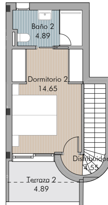
PLANTA PRIMERA
