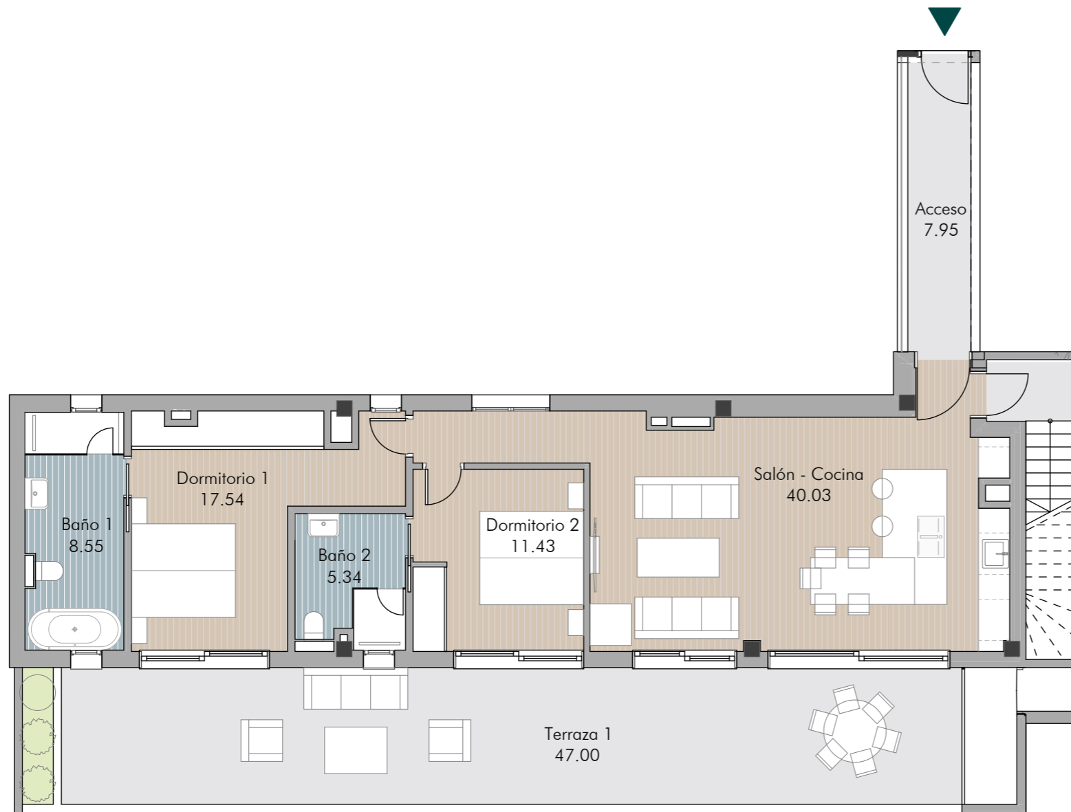
PLANTA SEGUNDA
