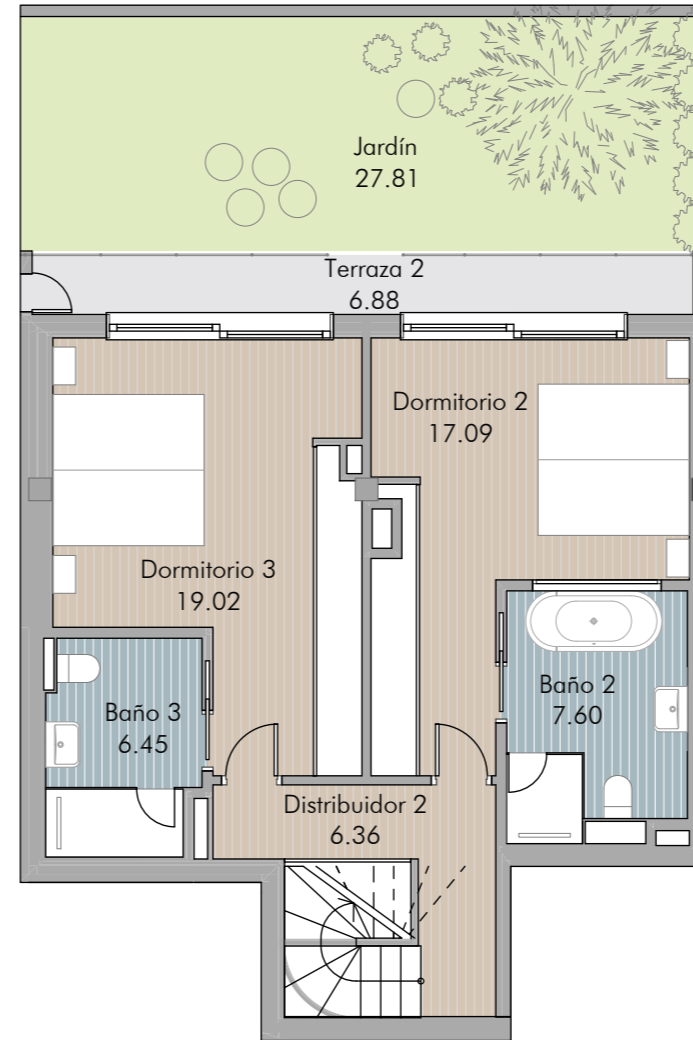
PLANTA SEGUNDA
