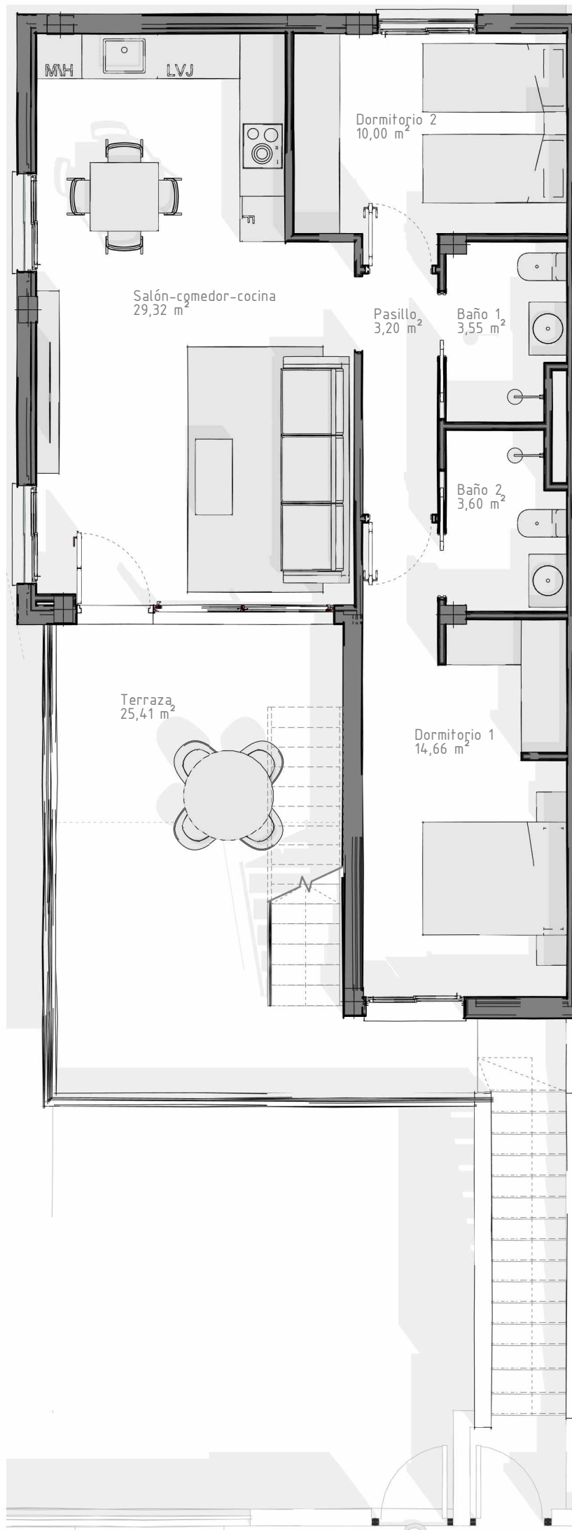
Planta alta
