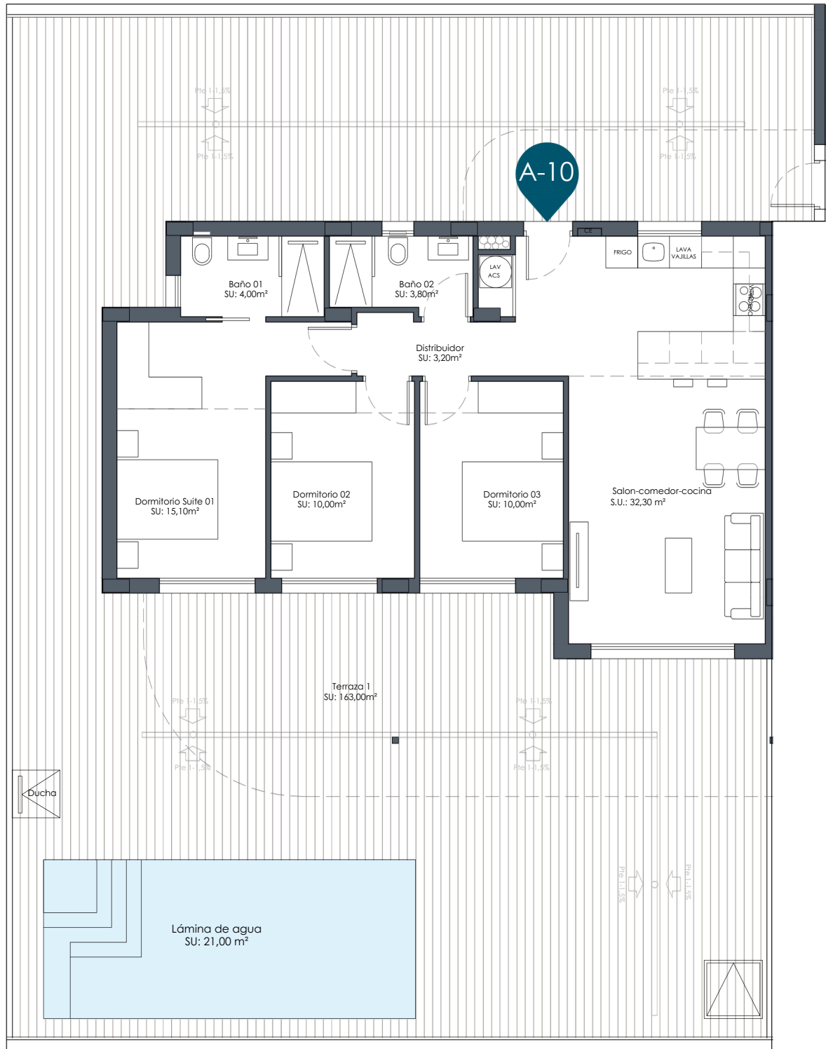
PLANTA BAJA
