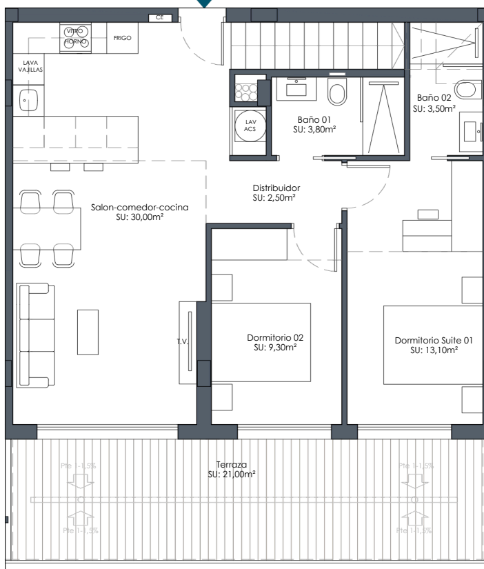
PLANTA SEGUNDA
