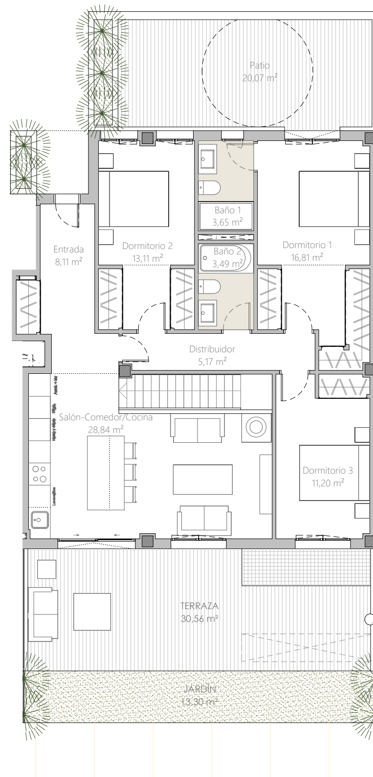
PLANTA BAJA
