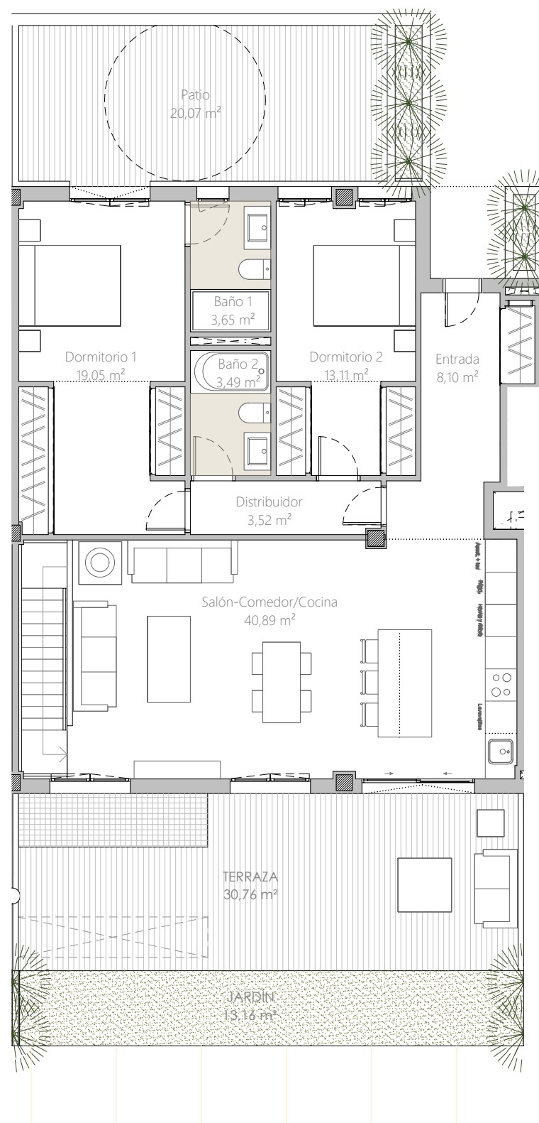
PLANTA BAJA
