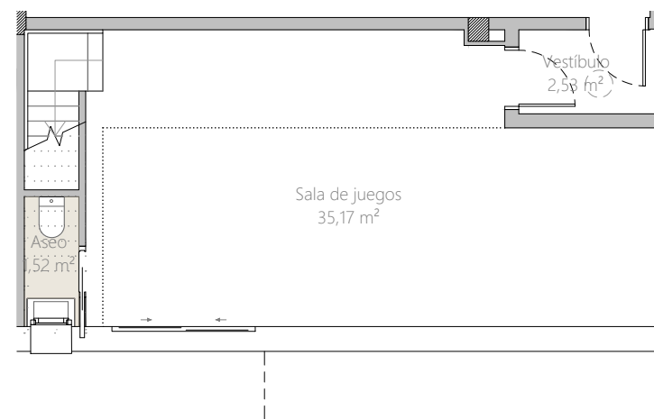
PLANTA SÓTANO
