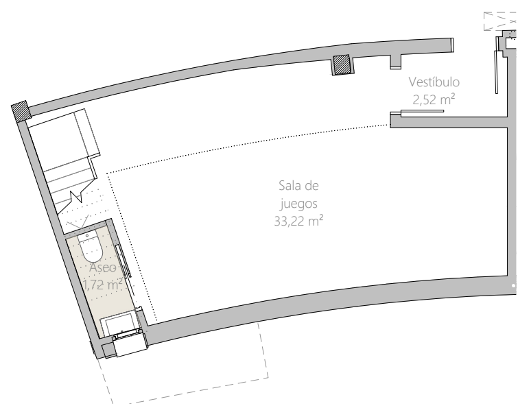
PLANTA SÓTANO
