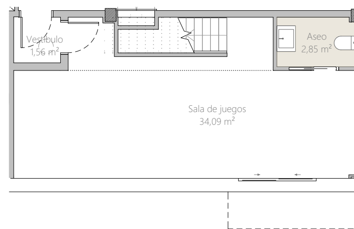
PLANTA SÓTANO
