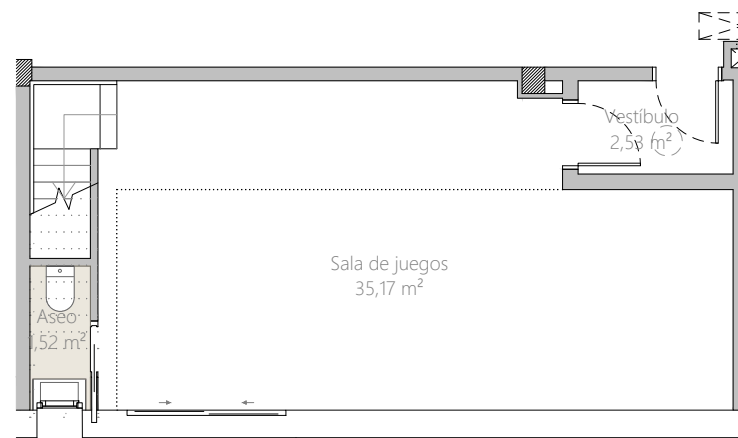
PLANTA SÓTANO
