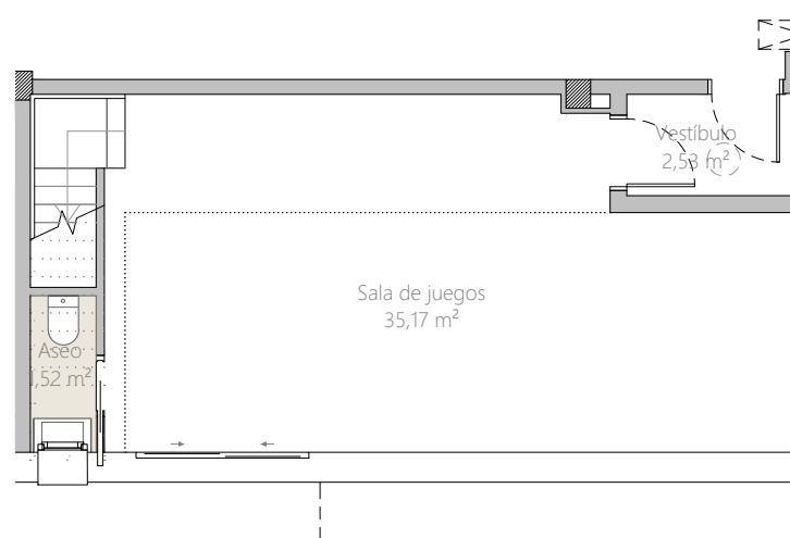
PLANTA SÓTANO
