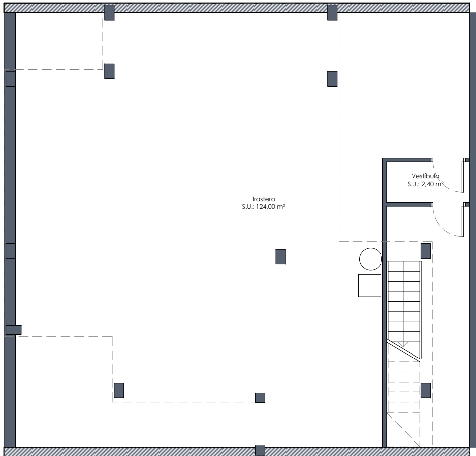
PLANTA SÓTANO
