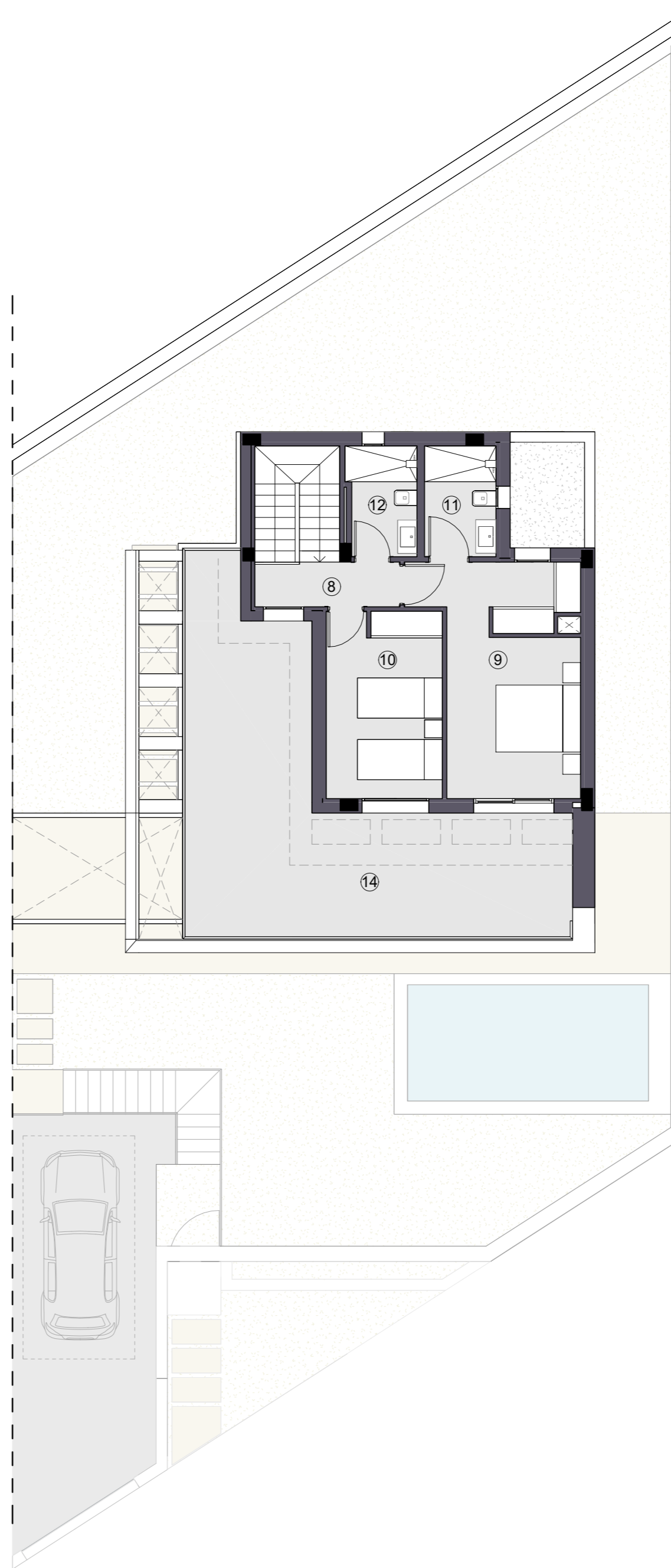
PLANTA PRIMERA / FIRST FLOOR
