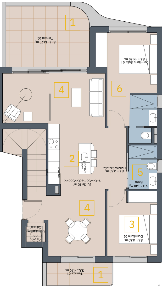
PLANTA SEGUNDA
