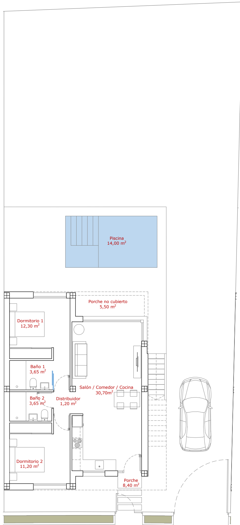
Planta Baja
