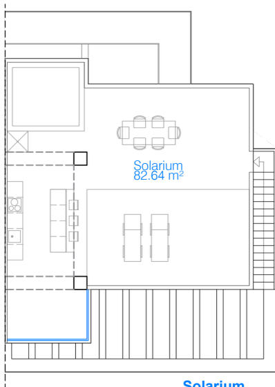
Solarium (E:1/200)
