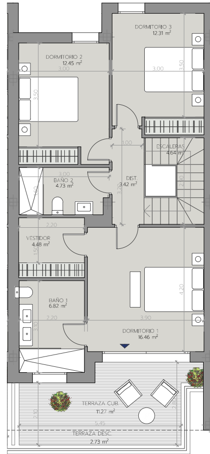
PLANTA PRIMERA
