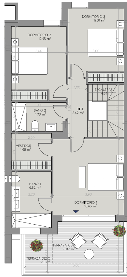
PLANTA PRIMERA
