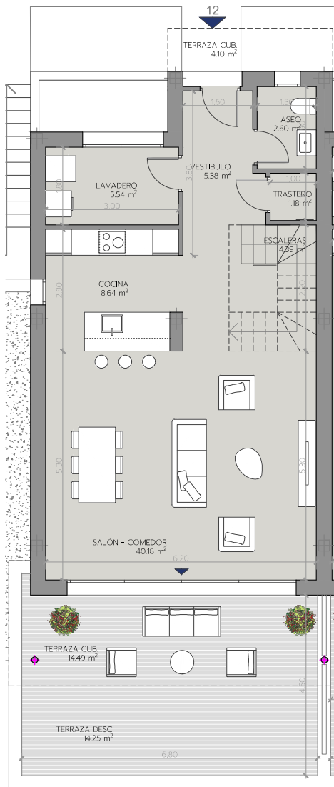
PLANTA BAJA
