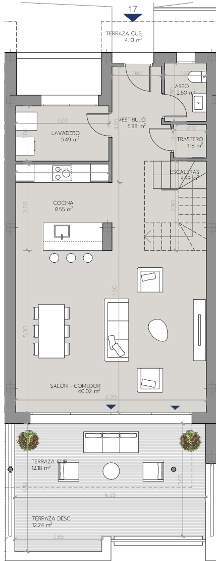
PLANTA BAJA
